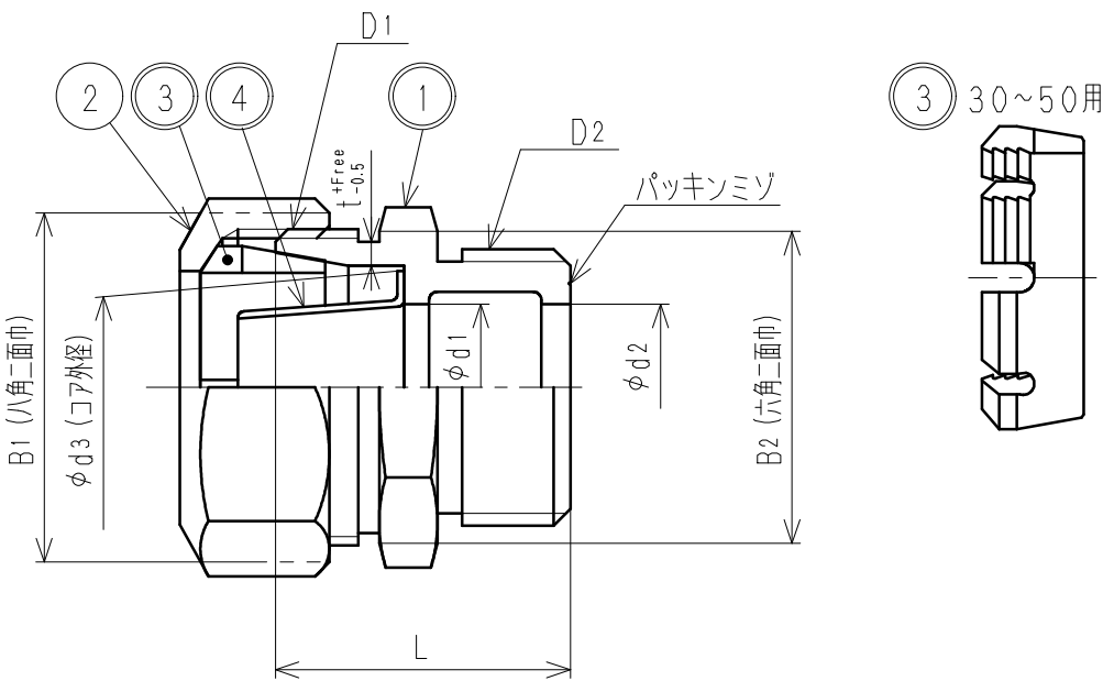
寸法表
